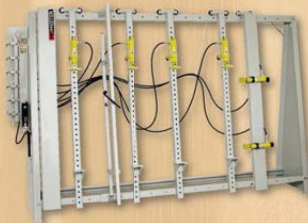
SLH 1 Frame hydraulic press Leimpresse SLH 1 Клеильный пресс SLH 1
